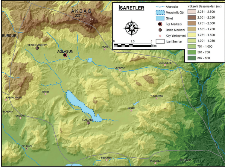
Şekil 2. Araştırma sahasının topografya haritası.
